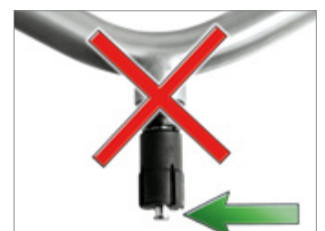
Spreizdübel zu weit eingedreht
