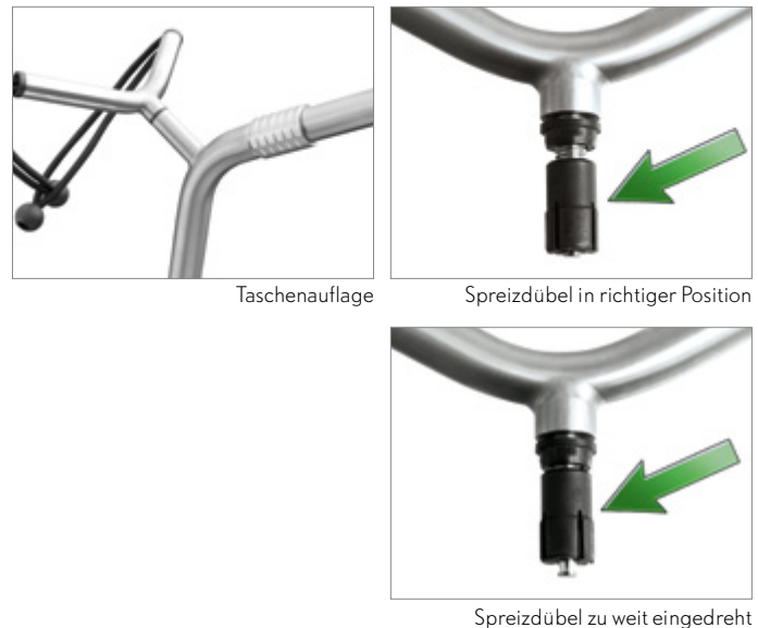
Spreizdübel zu weit eingedreht
